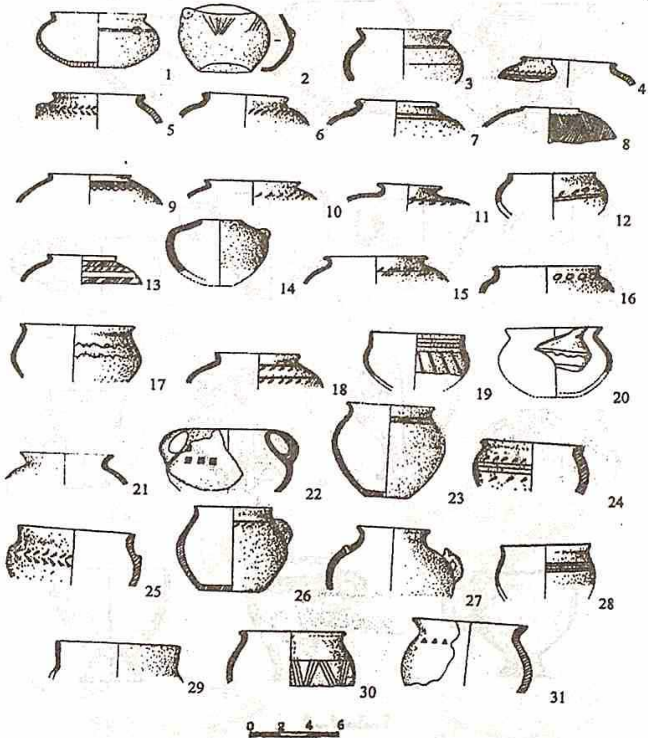
Şəkil 2. 19. Boz rəngli çölməklər: 1-3, 23-Boyəhməd nekropolu; 4, 5, 24, 25- Kolanı nekropolu; 6, 7-Qarnıyarıq yaşayış yeri; 8-11, 26,27-Haqqıxlıq nekropolu; 12-18, 28-Sarıdərə nekropolu; 19, 29-Qalacıq yaşayış yeri; 20-Kükü yaşayış yeri; 21-İlikliqaya yaşayış yeri; 22-Dəmyələr yaşayış yeri; 30-Şahtaxtı nekropolu; 31-İlikliqaya nekropolu.
