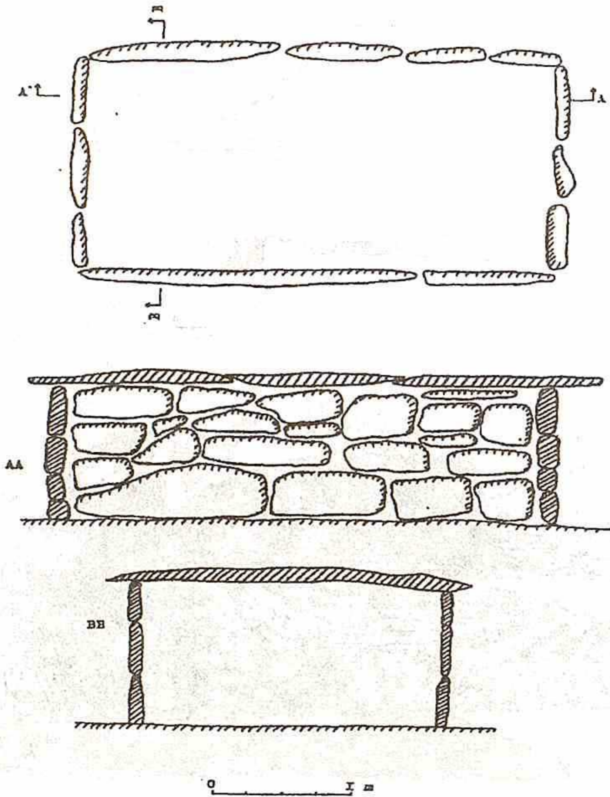
Şəkil 1. 6. Haqqıxlıq nekropolundakı 2 №-li qəbrin planı. (V.Baxşəliyev 2002).
