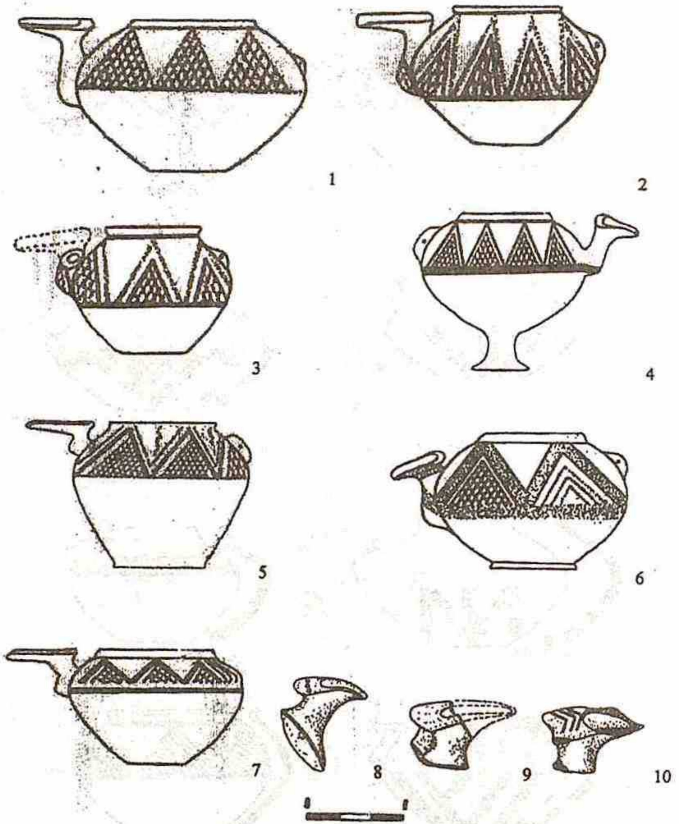
Şəkil 2. 26. Çayniklər: 1, 5, 7-Qızılburun nekropolu; 2, 3, 4-Naxçıvan nekropolu; 6-Şortəpə nekropolu; 8-İlikliqaya nekropolu; 9, 10-Sarıdərə nekropolu.
